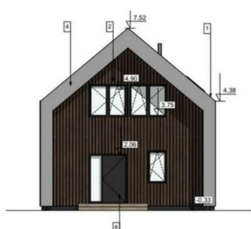
elewacja frontowa
