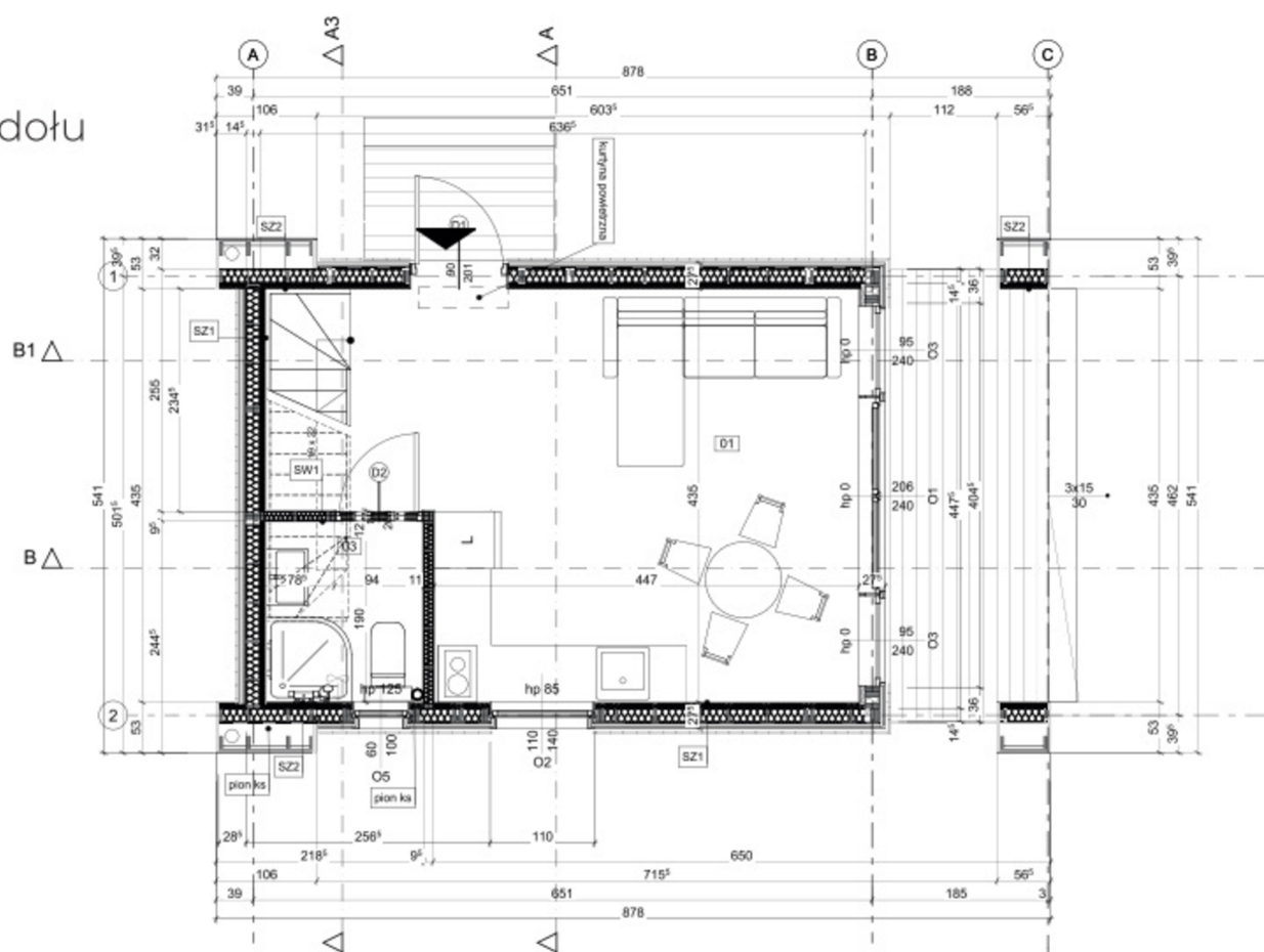
Rzut góry
